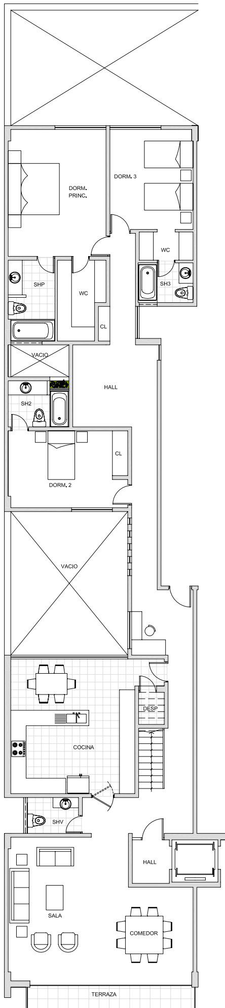
1º PISO DUPLEX 501 AREA TECHADA - 280.26 m 2 AREA OCUPADA - 412.31 m 2
